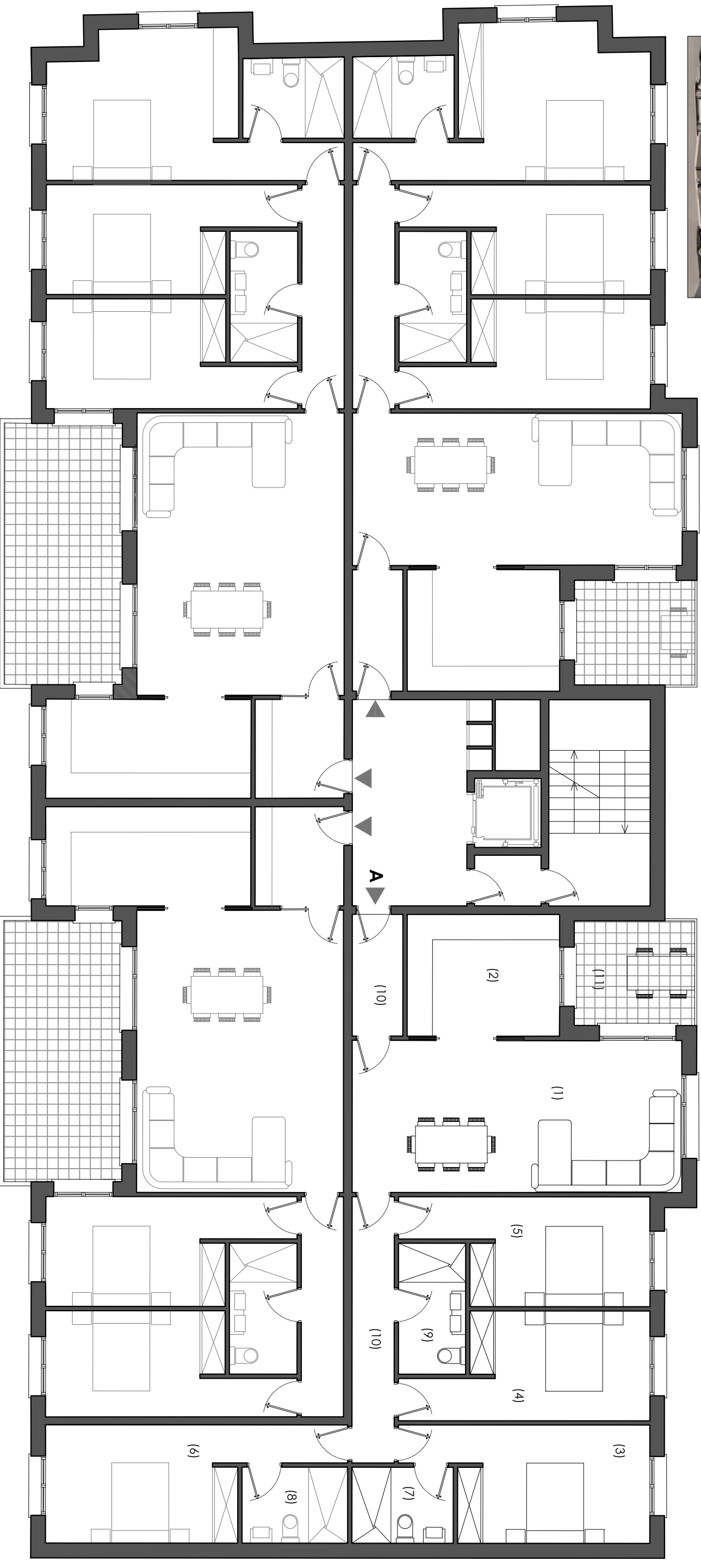
PLANTA PRIMERA Piso 1º A
